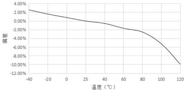
灵敏度温度响应曲线
